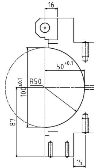
A-A SECTION
