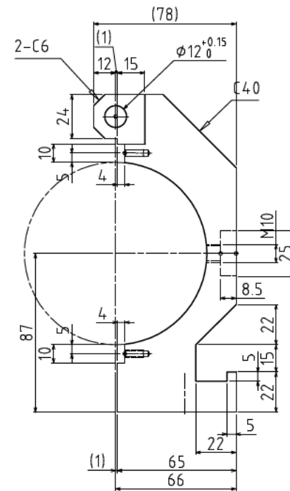
B'B SECTION
